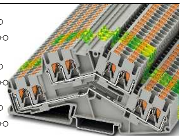
24 А, двухъярусная клемма, 4 разъема на ярус
