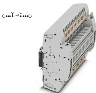
6 (10) мм 2 , 30 А, 4 ... 25-конт. контрольная колодка, установка на монтажную рейну, зажим push-in
