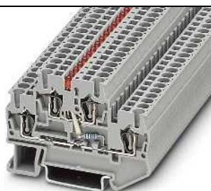
26 А, двухъярусная клемма со световым индикатором
