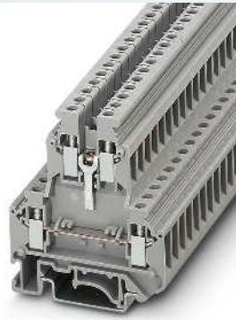
4 (4) мм 2 , 32 А, двухъярусная клемма с припайванием компонентов
