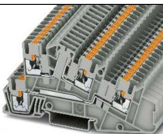
30 А, трехъярусная клемма, 1 внешний провод L, 1 раздельная зона
