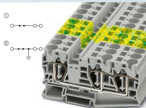
76 А, проходная клемма, 3 разъема
