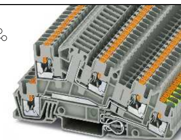
30 А, трехъярусная клемма, 1 внешний провод L, 1 PE, 1 раздельная зона
