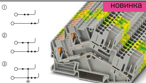
22 А, двухъярусная клемма, панельная конструкция
