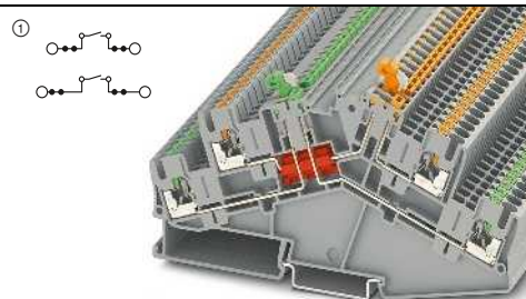
16 А, двухъярусная клемма с ножевым размыкателем на каждом ярусе, панельная конструкция
