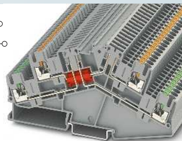
16 А, двухъярусная клемма с двумя раздельными зонами
