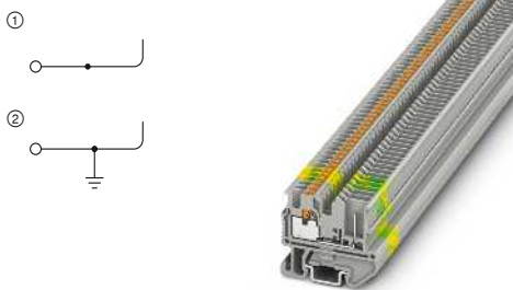
17,5 А, проходной блок мини-зажимов
