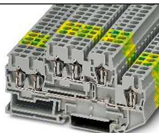
26 А, проходной блок зажимов, 3 разъема на каждом ярусе
