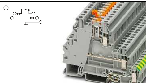
36 А, многоярусная клемма с ножевой раздельительной зоной, с основанием РЕ
