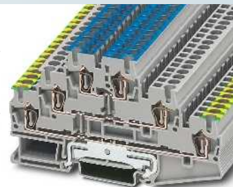
28 А, трехъярусная клемма с основанием PE
