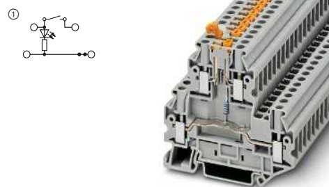
38 А, многоярусная клемма с ножевой раздельительной зоной, со световым индикатором
