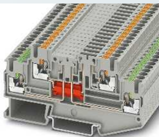
16 А, двухъярусная клемма с одной раздельной зоной
