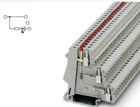
2,5 (4) мм 2 , 26 А, трехпроводная клемма со световым индикатором
