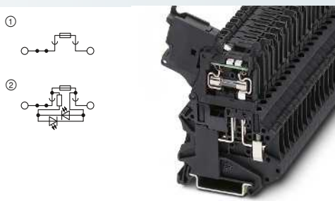
10 А, клемма рычажного предохранителя для стеклянных предохранителей 5 x 20 мм
