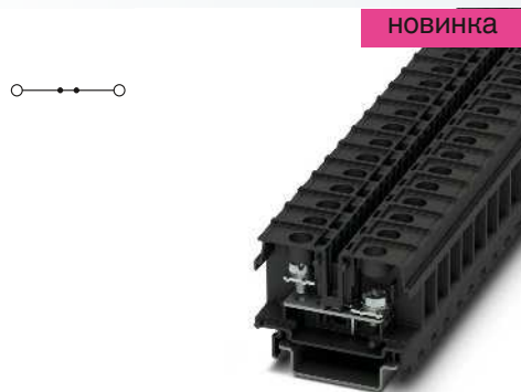
32 А, проходная клемма, закрытая
