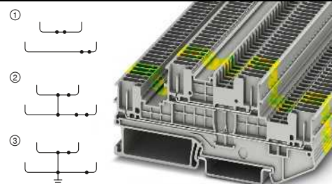
16 А, двухъярусные клеммы
