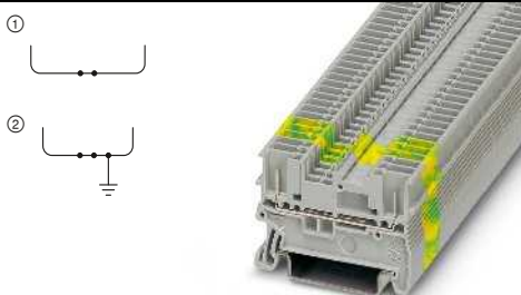
17,5 А, проходной блок зажимов
