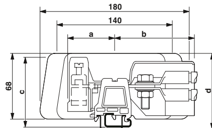
Размеры крышек и разделителей клеммных групп [мм] / [дюйм]
