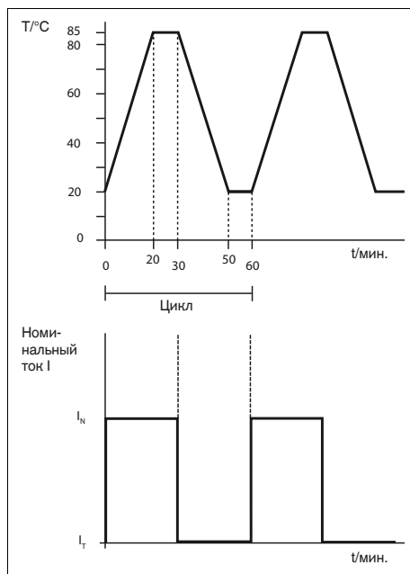
Ток и температура в зависимости от времени
