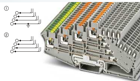
10 А, четырехъядрусная клемма с заземляющим основанием
