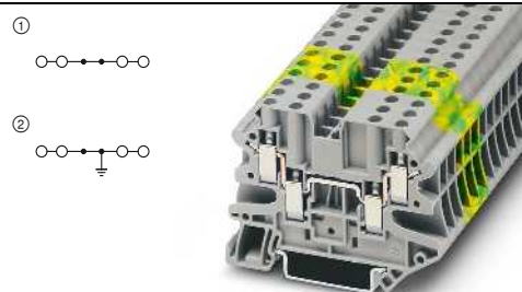
39 А, проходные и заземляющая клемма, 4 разъема
