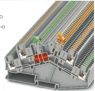
16 А, двухъярусная клемма с ножевым размыкателем на каждом ярусе, панельная конструкция
