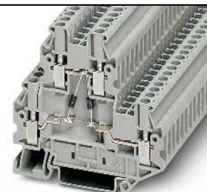
28 А, двухъярусная клемма с двумя диодами 1N 4007 (1300 В/0,5 А)
