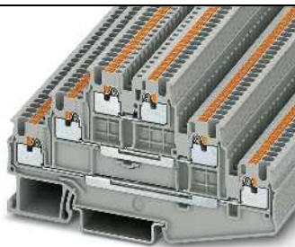
15 А, многоярусная клемма, 6 разъемов
