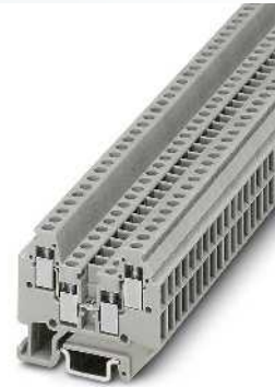
1,5 (1,5) мм 2 , 16 А, проходная клемма, 4 контакта
