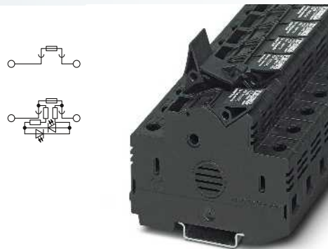
16 (25) мм 2 , 32 А, клемма рычажного предохранителя для малогабаритного плавкого предохранителя 10,3 x 38 мм
