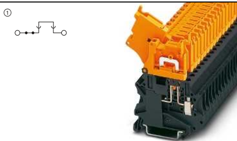
20 А, клемма с рычажным размыкателем, той же формы
