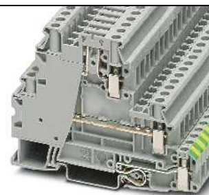
36 А, многоярусная клемма с разделительной зоной и основанием PE
