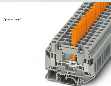
6 (10) мм 2 , 57 А, разделительная клемма
