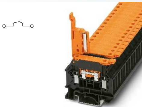
4 (6) мм 2 , 16 А, рычажная разделительная клемма, той же формы
