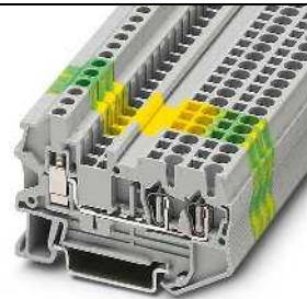
28 А, проходной блок зажимов, 3 разъема
