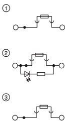
10 А, клемма с держателем предохранителя (для стеклянных предохранителей) 5 x 20 мм
