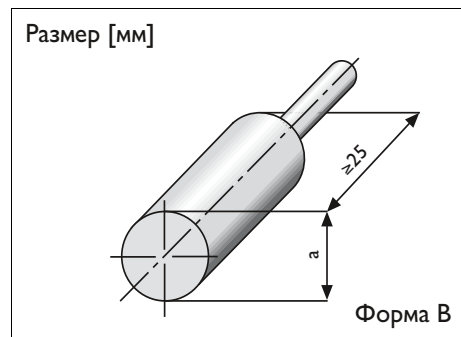
Шаблоны (калибровочные пробки) форм А и В согласно МЭК 60947-1
