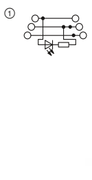
28 А, трехъярусная клемма со световым индикатором
