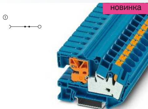
68 А, разделительная клемма N
