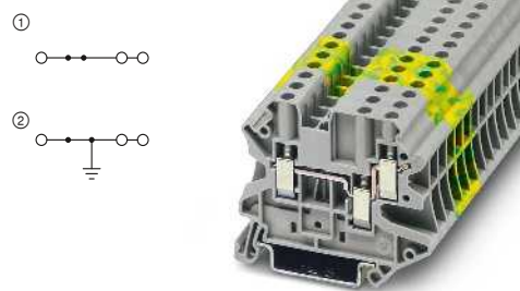
41 А, проходные и заземляющие клеммы, 3 разъема
