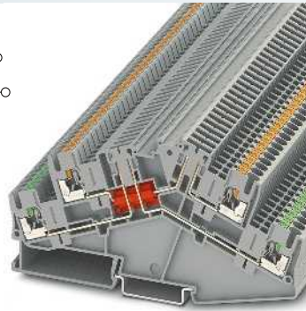
16 А, двухъярусная клемма с двумя разделительными зонами
