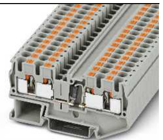
1,5 А, диодная клемма, 1N 5408 (1000 В/1,5 А)
