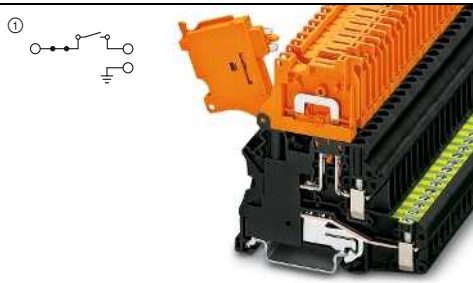
20 А, клемма с рычажным размыкателем, той же формы, с основанием PE
