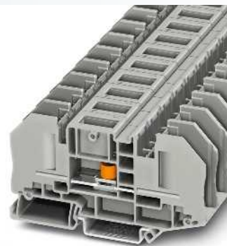
41 А, разделит. клемма для измерит. преобразователя, открытая
