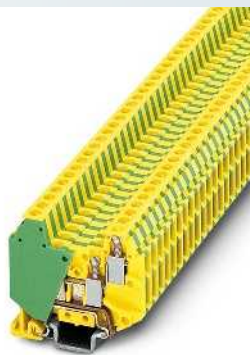
1,5 (1,5) мм 2 , заземляющая клемма, 4 разъема
