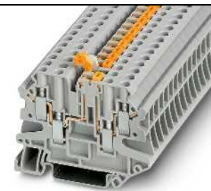
20 А, клемма с ножевым размыкателем, 4 разъема
