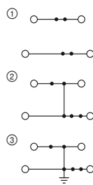
28 А, двухъярусная клемма
