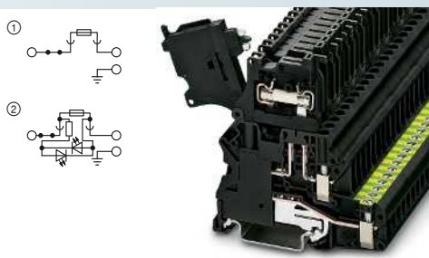
6,3 А, клемма рычажного предохранителя для стеклянных предохранителей 5 x 20 мм, с основанием PE
