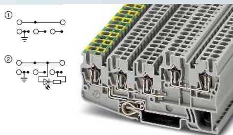
18 А, четырехпроводная клемма для исп. элемента с основанием PE
