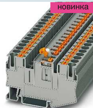
20 А, клемма с ножевым размыкателем
