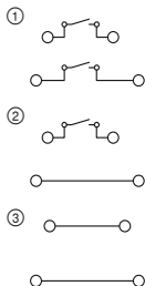
16 А, двухъярусная клемма с ножевым размыкателем на каждом ярусе
