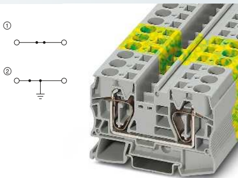
90 А, проходной блок зажимов
