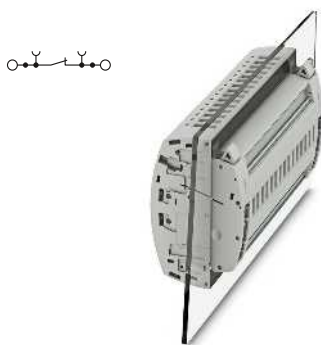
10 (10) мм 2 , 30 А, 4 ... 25-конт. контрольная колодка, для настенного монтажа, винтовой зажим
