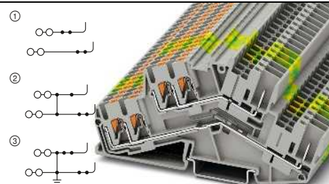
18 А, двухъярусная клемма, панельная конструкция
