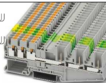
24 А, проходной блок зажимов, 6 разъемов
