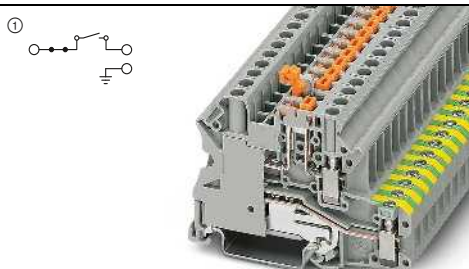
20 А, клемма с ножевым размыкателем и заземляющим основанием
