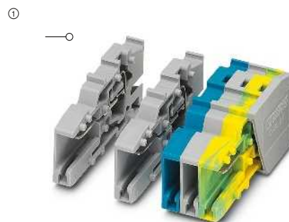
24 А, устройство сопряжения, самостоятельная сборка
