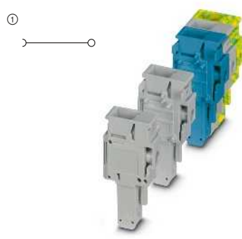
41 А, штекер, подключение в направлении вставления, для монтажа по месту
