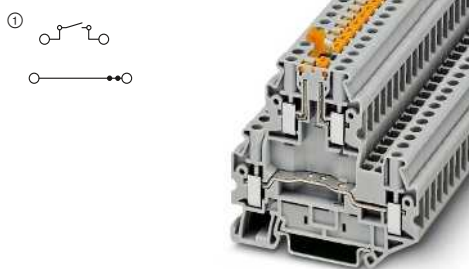
38 А, двухъярусная клемма с ножевой раздельительной зоной
