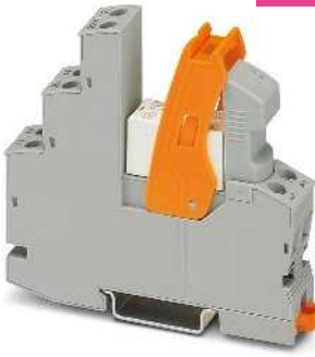
Релейный модуль с 2 переключающими контактами с винтовым зажимом
