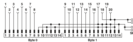
Схема подключения FLKM 14-PA-MODI/M340
