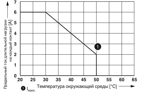
Кривая изменения состояний контакта
