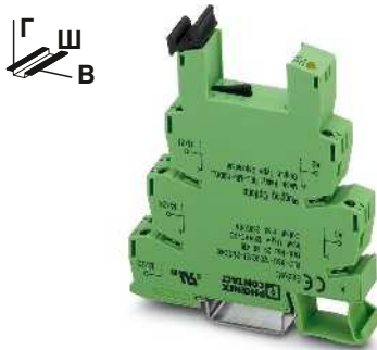
Базовая клемма с 2 переключающими контактами с входным фильтром
