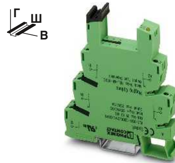
Базовая клемма с 1 переключающим контактом для повышенного тона длительной нагрузки с входным фильтром
